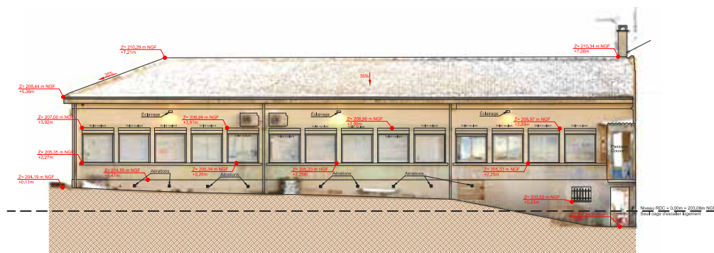
Réalisation des plans (niveaux, façades, coupes) : école de Mirabel.
